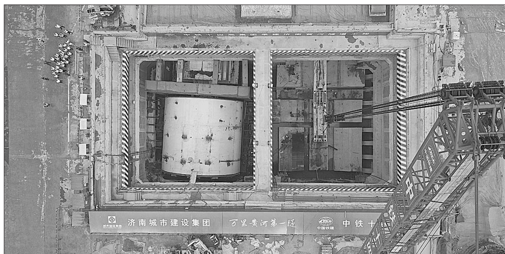
黄河隧道盾构机正加紧组装调试。
